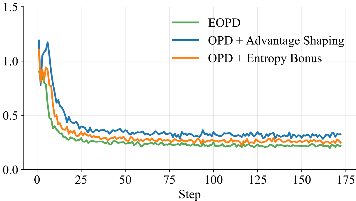
Forward KL Divergence
